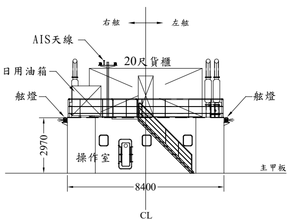
甲板室正視圖
